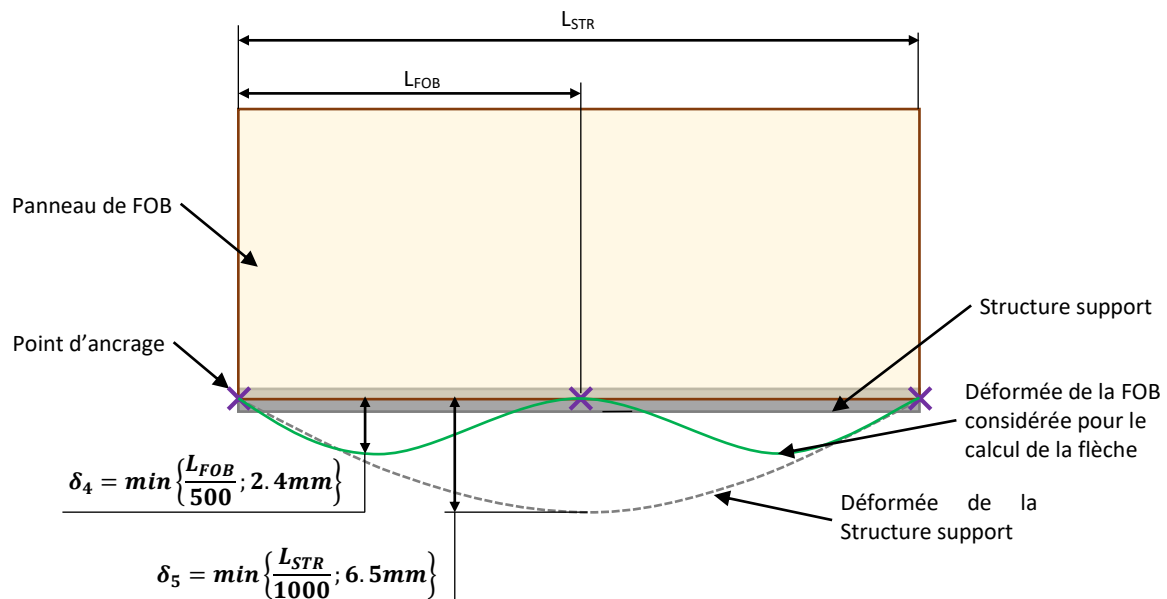
Figure 7 – Exemple de représentation du critère de flèche nuisible à respecter pour une FOB filante avec ancrage multiples sur poutres ou dalle – Configuration 1
