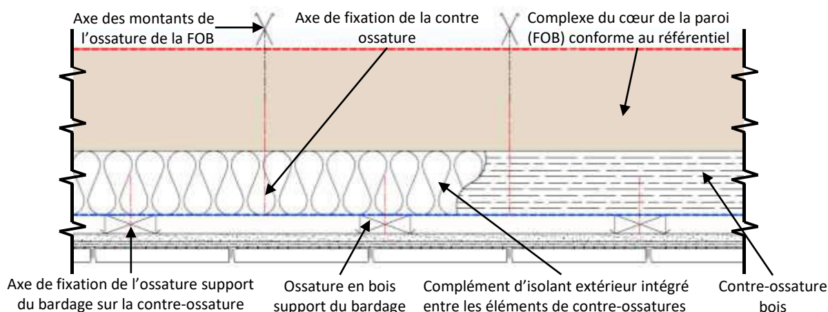
Figure 2 – Représentation de l'ossature simple réseau avec complément d'isolation par l'extérieur en coupe horizontale
