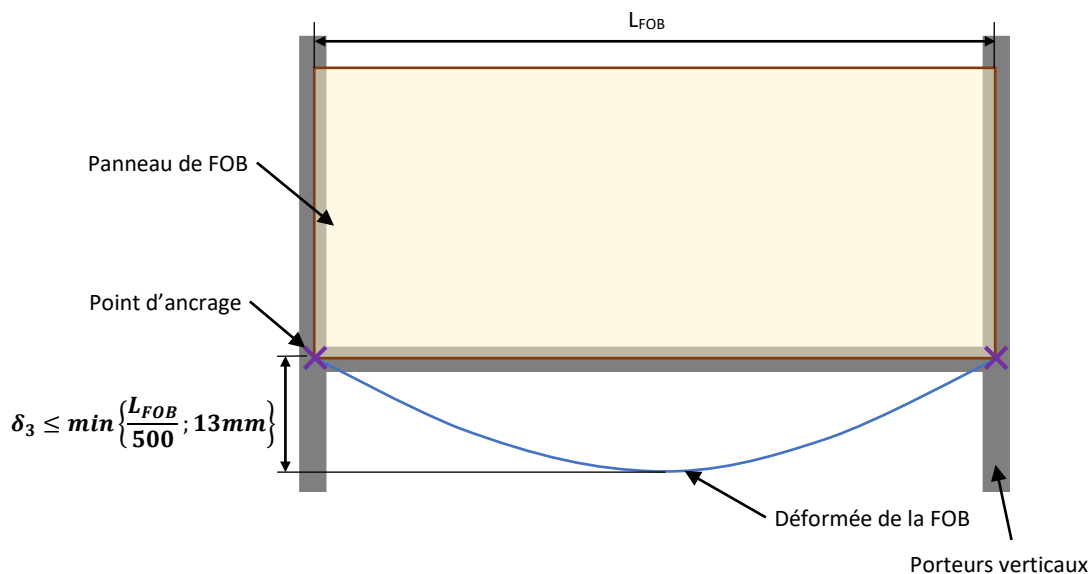
Figure 5 – Exemple de représentation du critère de flèche nuisible à respecter pour une FOB filante avec ancrage multiples sur porteurs verticaux – fonctionnement isostatique
