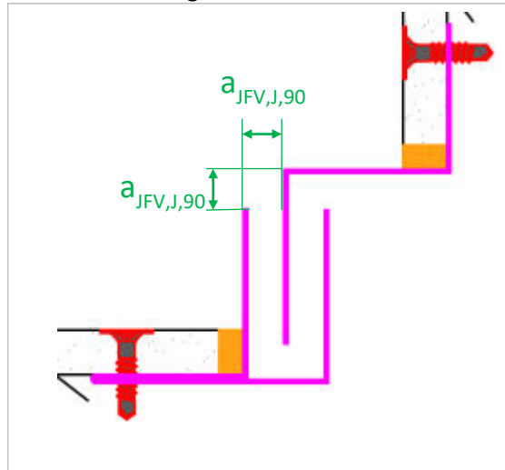
Figure 29 – Aperçu de la solution « d » Aperçu du traitement des jeux fonctionnels verticaux en angle rentrant
