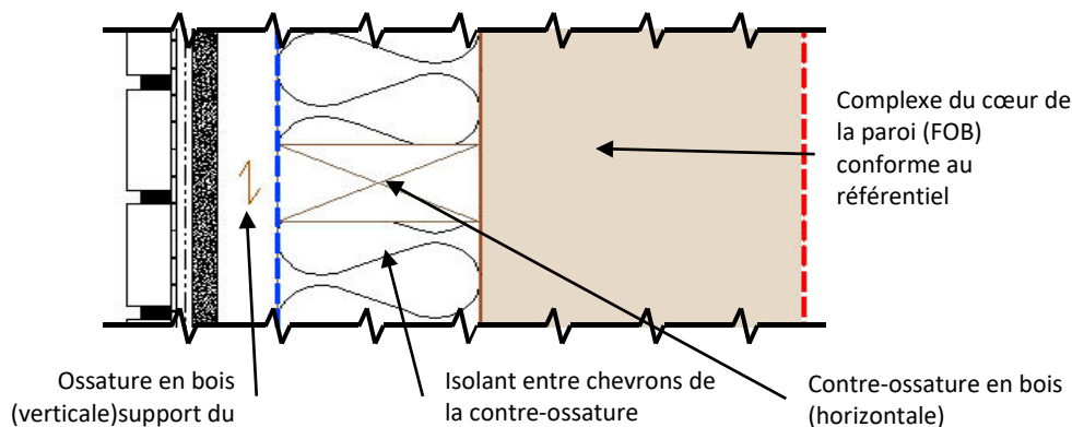
Figure 3 – Représentation de l'ossature simple réseau avec complément d'isolation par l'extérieur en coupe verticale
