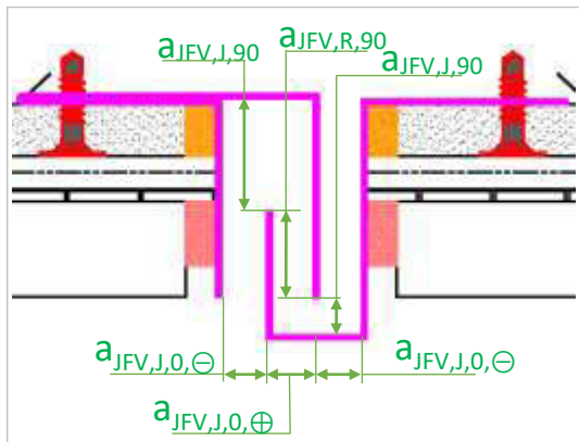
Figure 11 – Aperçu de la solution « a » pour le traitement des jeux fonctionnels verticaux
