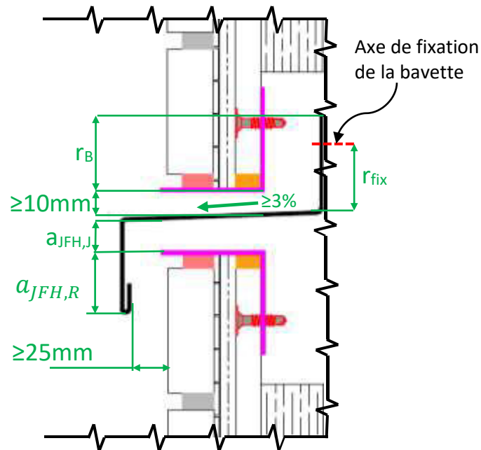
Figure 18 – cotes appliquées à la bavette et au bardage cas d'un revêtement collé
