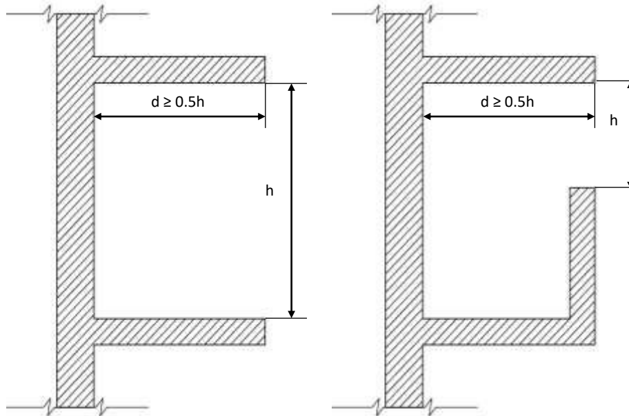
Figure 36 – Définition des éléments architecturaux de protection
