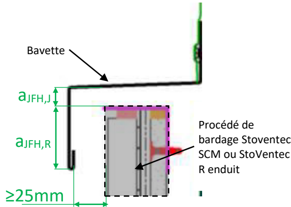
Figure 10 – Fixation de la bavette et conditions de forme
