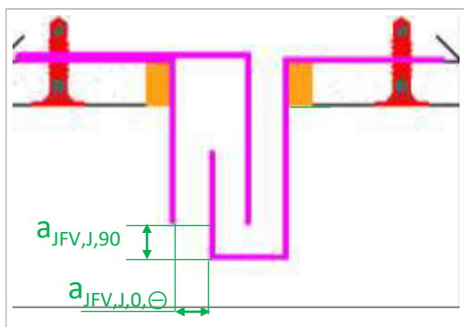
Figure 21 – Aperçu de la solution « a » pour le traitement des jeux fonctionnels verticaux (le revêtement de finition et la jonction avec le profil ne sont pas représentés, voir le §6.4 pour le traitement de cette jonction)
