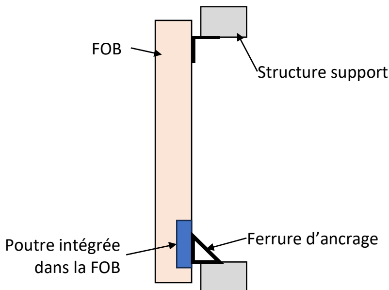
Figure 15 – Principe de poutre intégrée à la FOB (Coupe verticale)
