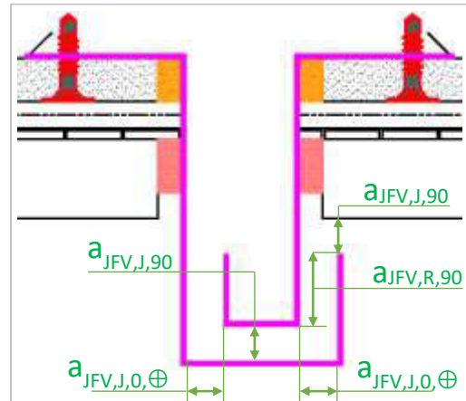
Figure 12 – Aperçu de la solution « b » pour le traitement des jeux fonctionnels verticaux
