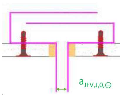
Figure 23 – Aperçu de la solution « c » pour le traitement des jeux fonctionnels verticaux (le revêtement de finition et la jonction avec le profil ne sont pas représentés, voir le §6.4 pour le traitement de cette jonction)
