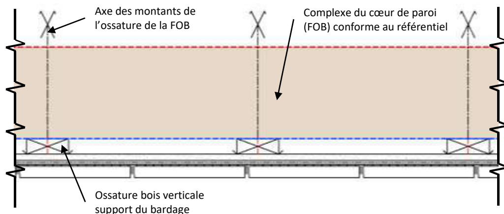
Figure 1 – Représentation de l'ossature Simple réseau en coupe horizontale
