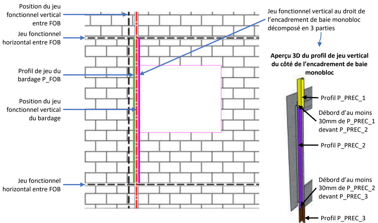
Figure 25- Elévation d'un jeu fonctionnel Vertical au droit d'une baie
