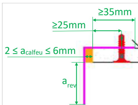
Figure 16 – Aperçu du traitement des extrémités des StoPanneaux Ventec – cas d'une cornière
