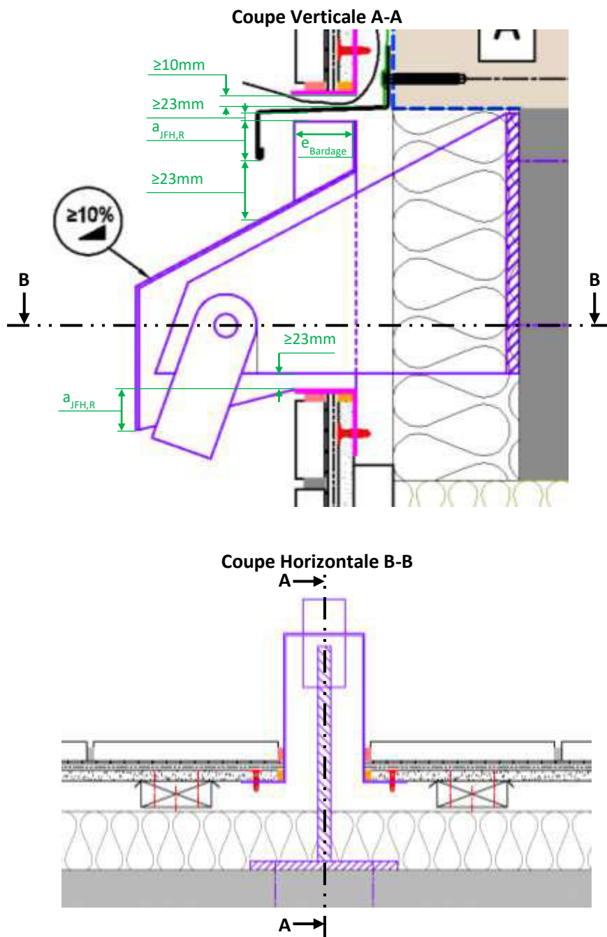
Figure 34 – Exemple de traitement de la continuité de l'étanchéité à l'eau au niveau du bardage d'un élément ancré dans la structure en traversant le bardage mais sans traverser la FOB
