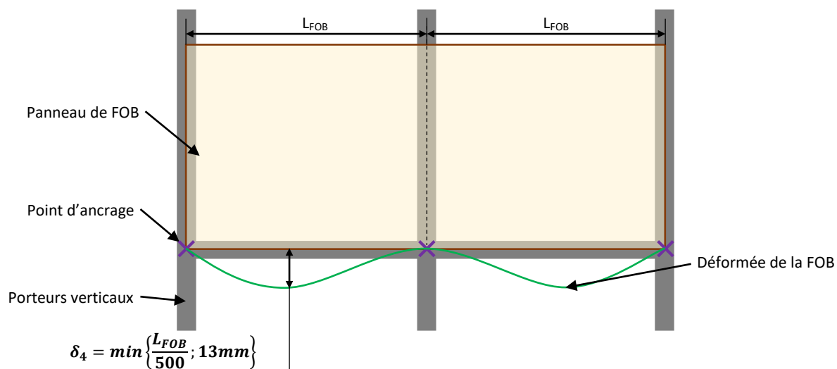
Figure 5 – Exemple de représentation du critère de flèche nuisible à respecter pour une FOB filante avec ancrage multiples sur porteurs verticaux – fonctionnement isostatique
