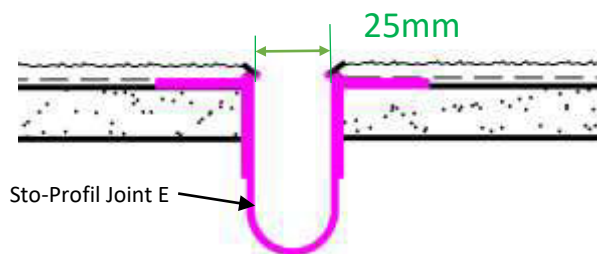
Figure 24 – Aperçu de la solution « d » pour le traitement des jeux fonctionnels verticaux
