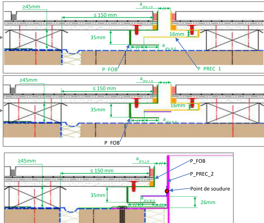
Figure 27- Coupes horizontales sur le jeu fonctionnel (1/2)
