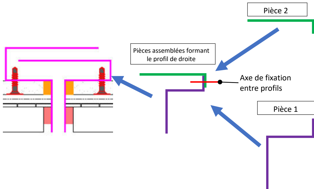
Figure 20 – Principe d'assemblage d'un profil de jeu fonctionnel creux réalisé en 2 pièces
