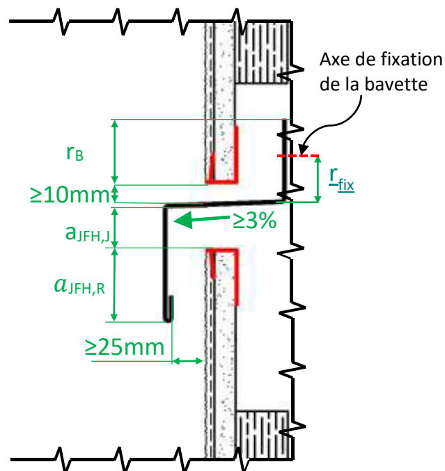
Figure 19 – cotes appliquées à la bavette et au bardage cas d'une finition enduite
