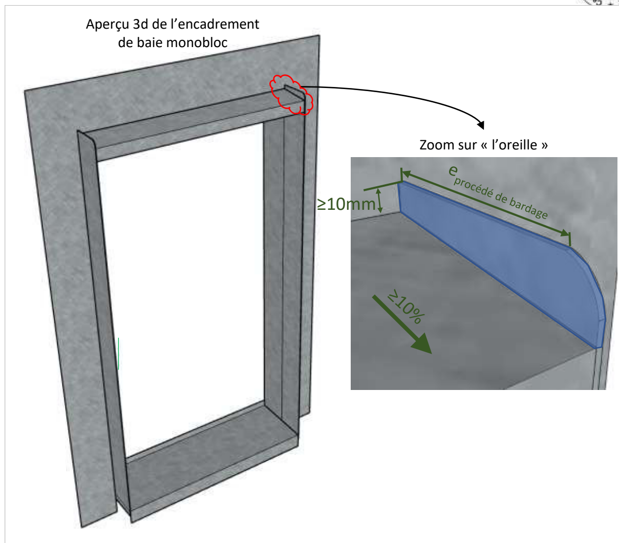
Figure 31 – Aperçu 3d du traitement de « l'oreille » en linteau de l'encadrement de baie monobloc
