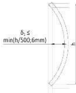
Figure 4 - Représentation du déplacement limite hors plan
