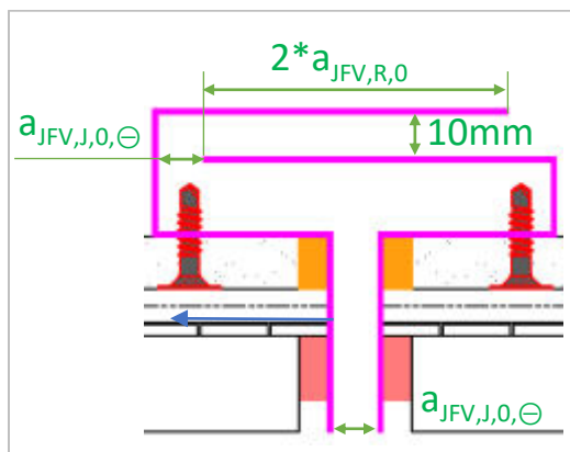
Figure 13 – Aperçu de la solution « c » pour le traitement des jeux fonctionnels verticaux
