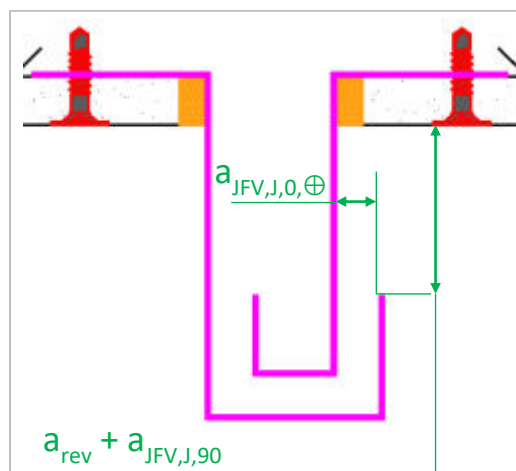
Figure 22 – Aperçu de la solution « b » pour le traitement des jeux fonctionnels verticaux (le revêtement de finition et la jonction avec le profil ne sont pas représentés, voir le §6.4 pour le traitement de cette jonction)
