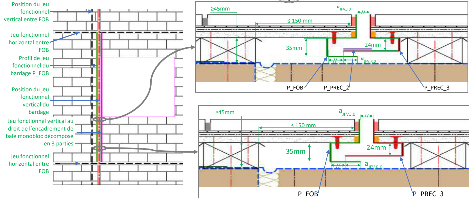
Figure 28- Coupes horizontales sur le jeu fonctionnel (2/2)
