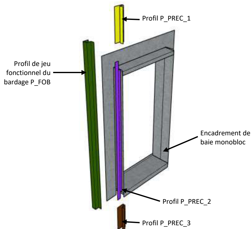
Figure 26- Aperçu 3D des éléments constituant le jeu fonctionnel
