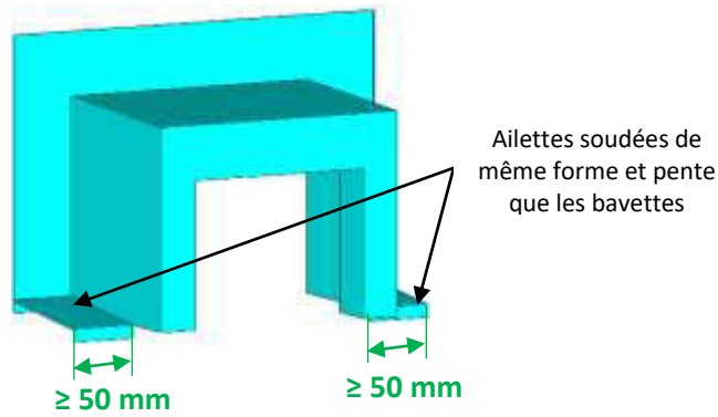
Figure 33 – exemple d'un aperçu 3D de la pièce monobloc étanche supérieure avec des ailettes pour faire la jonction avec un jeu fonctionnel horizontal avec bavette
