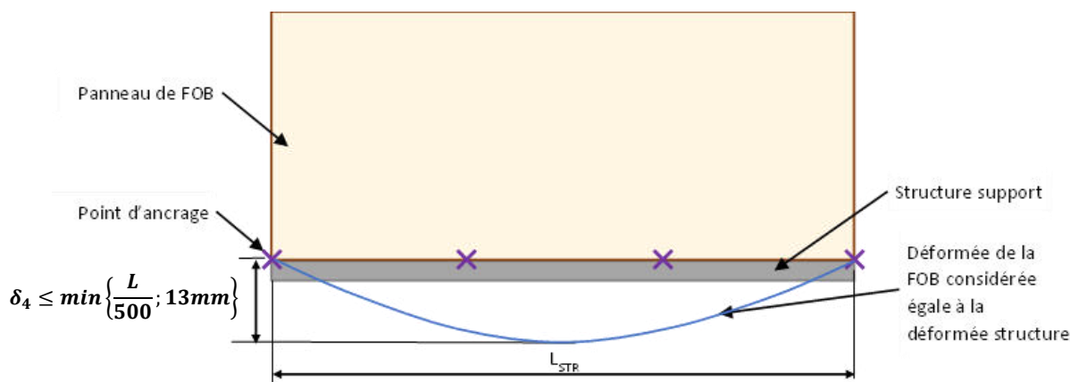
Figure 9 – Représentation du critère de flèche nuisible à respecter pour une FOB interrompue (NB : les déformées sont représentées de façon volontairement exagérée)
