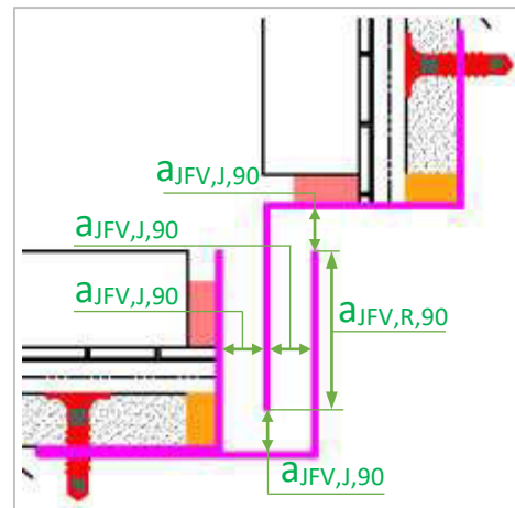
Figure 14 – Aperçu de la solution « d » pour le traitement des jeux fonctionnels verticaux en angle rentrant
