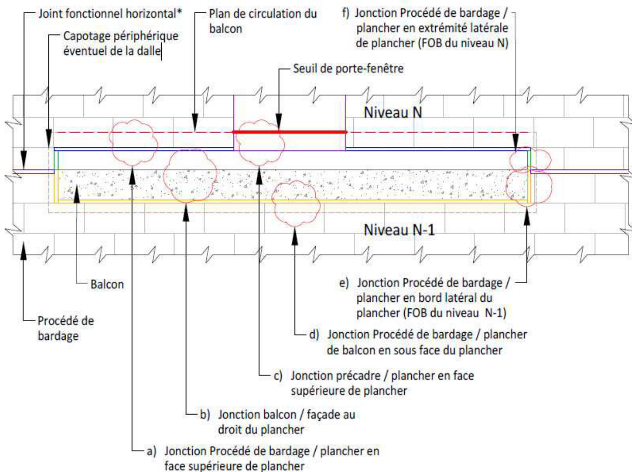
Figure 32 – Aperçu des jonctions du procédé de bardage / balcon ou coursive sur une élévation
