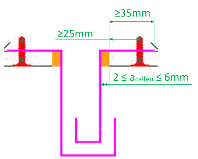
Figure 17 – Aperçu du traitement des extrémités des StoPanneaux Ventec – exemple pour un profil de jeu fonctionnel saillant
