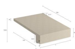
StoDeco Frame F type AF P.395
