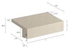
StoDeco Frame F type AF P.495
