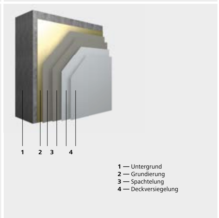
Aufbau des Cleanroom Wall/Ceiling Systems (Beispiel)
