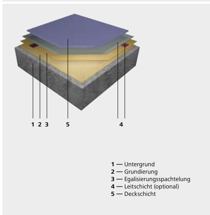
Aufbau des StoFloor Cleanroom Systems (Beispiel)
